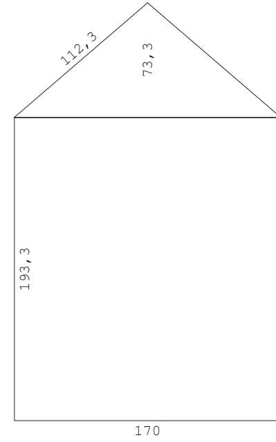
Profil droit
